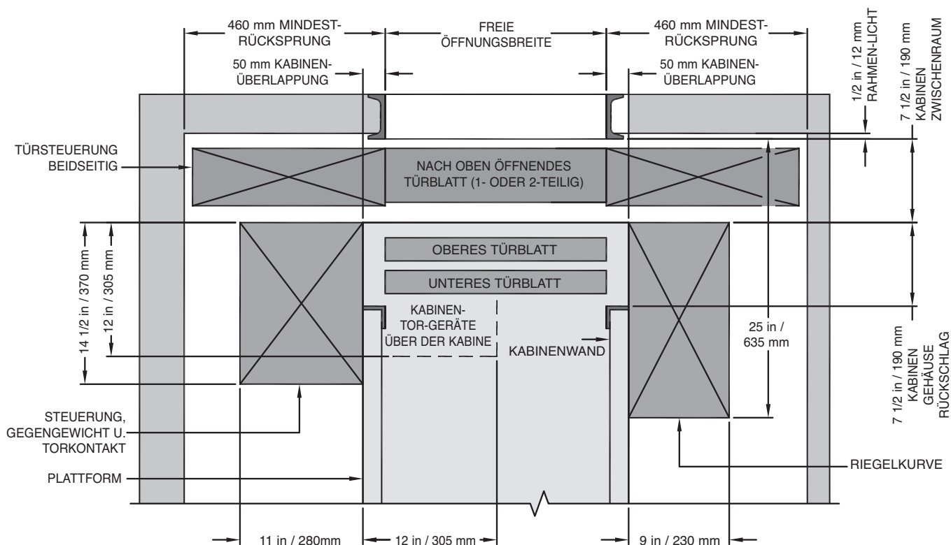
SCHNITTDRAUFSICHT
