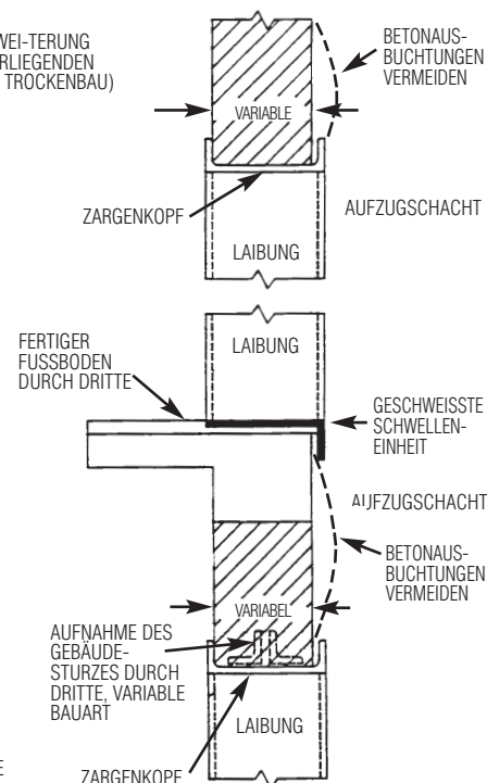
VERTIKALER QUERSCHNITT VON RAHMEN UND SCHWELLE DURCH DIE ÖFFNUNG
