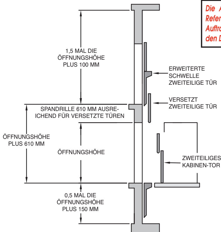
SCHNITTANSICHT - VERTIKALEN ABMESSUNGEN
