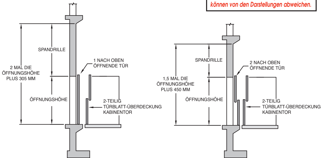
SCHNITTANSICHT - VERTIKALEN ABMESSUNGEN
