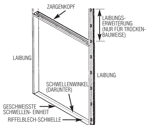
U-STAHL-TÜRZARGE
