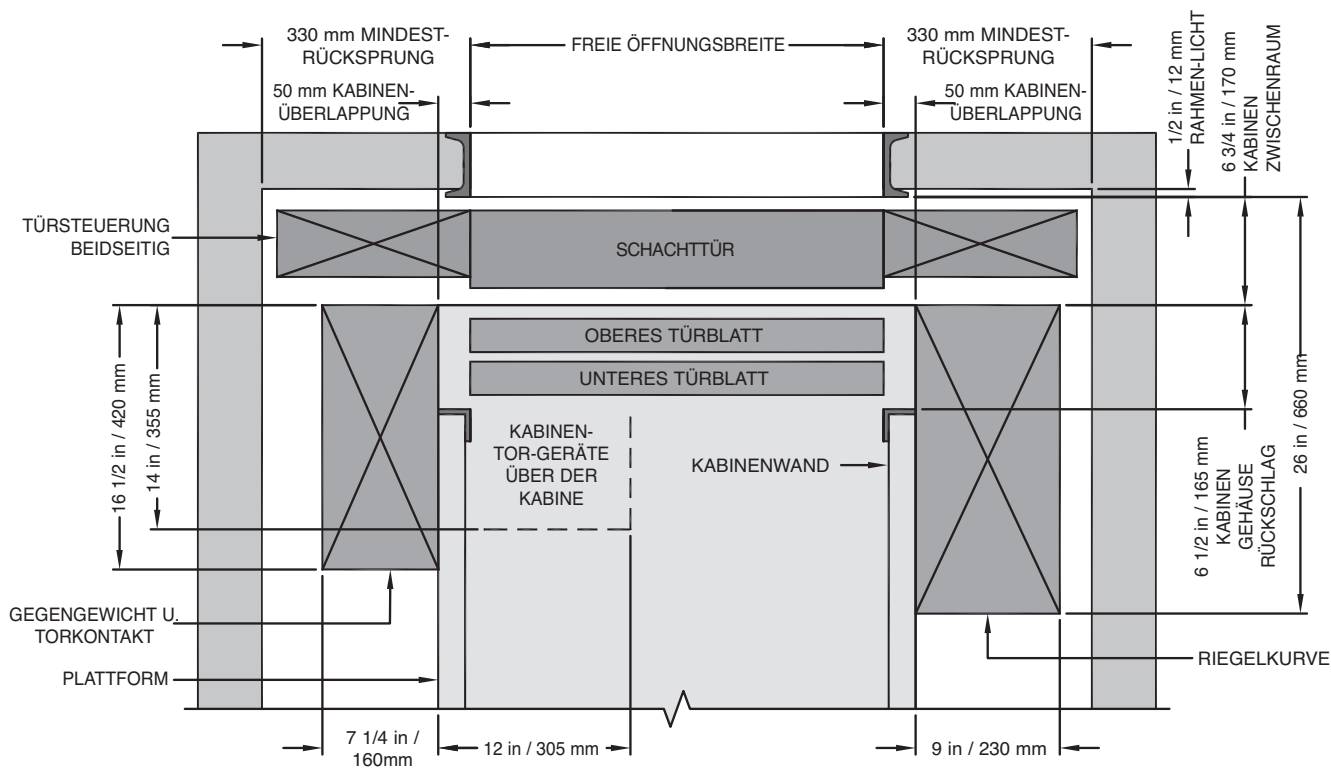
SCHNITTDRAUFSICHT
