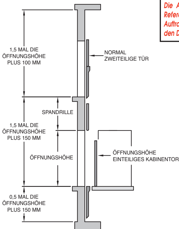
SCHNITTANSICHT - VERTIKALEN ABMESSUNGEN
