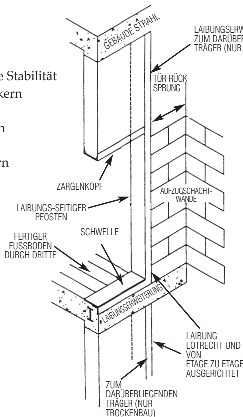
ANSICHT VOM AUFZUGSCHACHT
