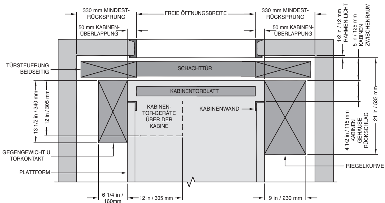
SCHNITTDRAUFSICHT
